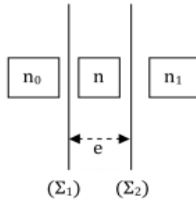
Cas dissymétrique : lame n_0/n/n_1
