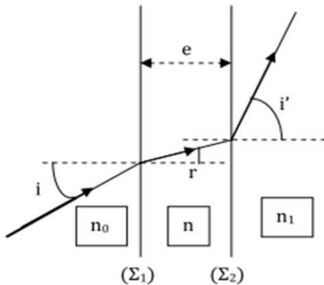
Cas dissymétrique : lame n_0/n/n_1
