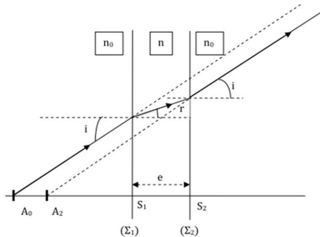
Cas symétrique : lame n_0/n/n_0
